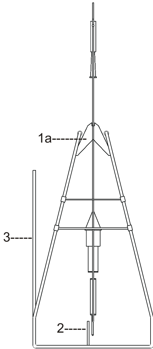
Side Elev.
